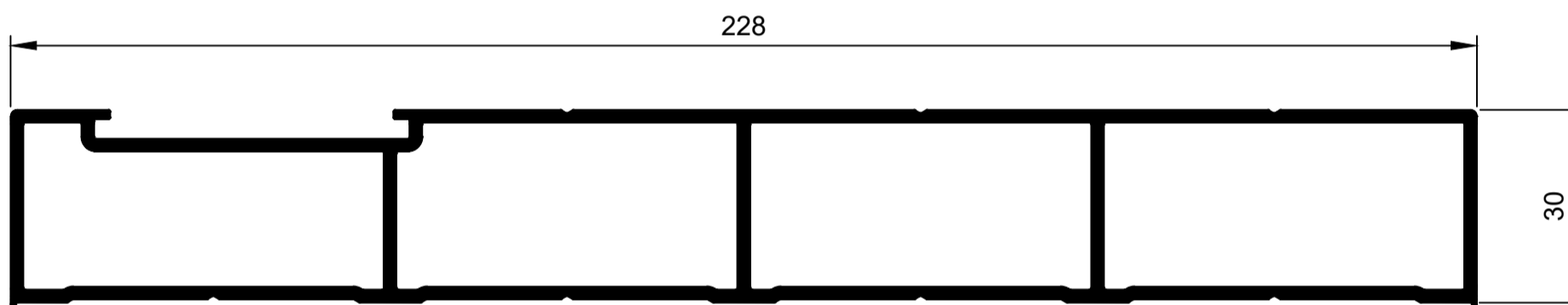
KSD005 Jamb Quadruple KELL Ix: 572.726cm 4
